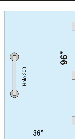
Only Door--3x8 ft
